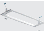
ZESTAW DO MONTAŻU DOSTROPEWEGO Wycięcie montażowe 414X150 mm
