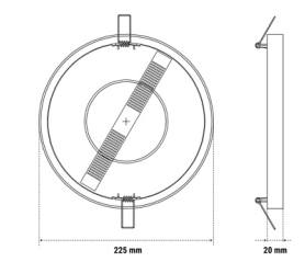
Foro di ingresso Ø 65-210 mm
