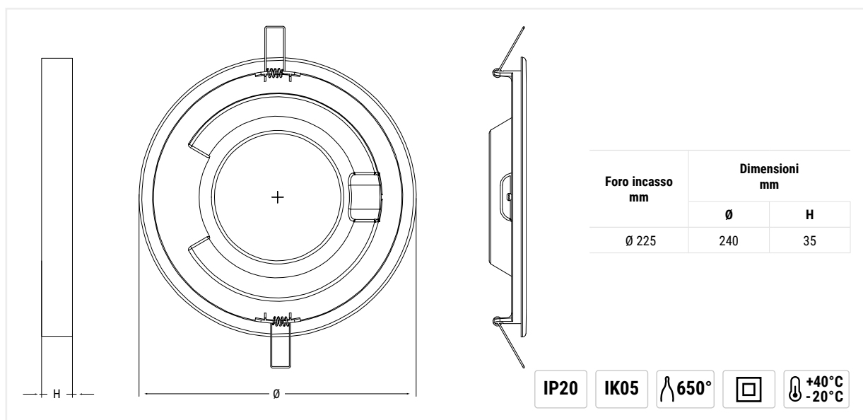
Molle per installazione a incasso controsoffitto - 2 pezzi
