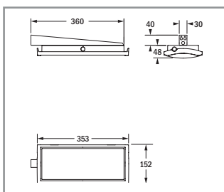
Výložník (37093, 37094, 37095, 19296, R2436SA)
